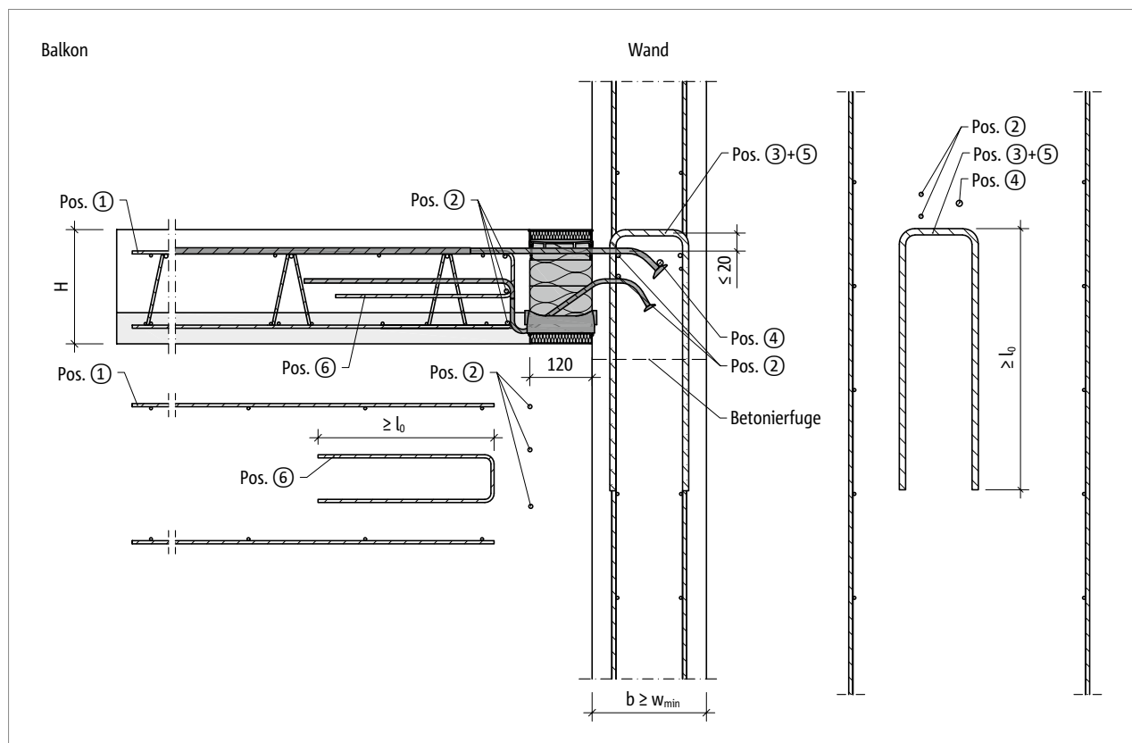
Abb. 129: Schöck Isokorb® XT Typ K-O-F: Bauseitige Bewehrung für Wandanschluss nach unten
