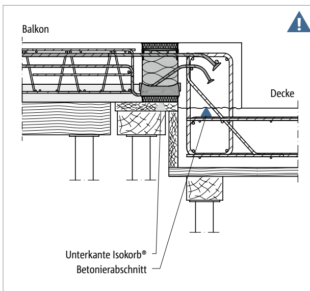
Abb. 133: Schöck Isokorb® XT Typ K-O-F: Halbfertigteilbalkon mit Höhenversatz nach oben
