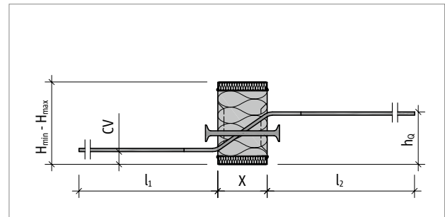
Abb. 193: Schöck Isokorb® XT Typ Q-P-V5 bis V16: Produktschnitt
