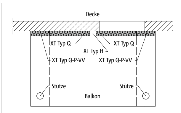
Abb. 179: Schöck Isokorb® XT Typ Q-P-VV, Q: Balkon mit Stützenlagerung bei unterschiedlichen Auflagersteifigkeiten; optional mit XT Typ HP
