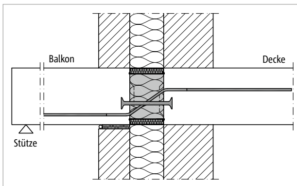
Abb. 181: Schöck Isokorb® XT Typ Q-P-V5 bis V16: Anschluss gestützter Balkon bei zweischaligem Mauerwerk mit Kerndämmung
