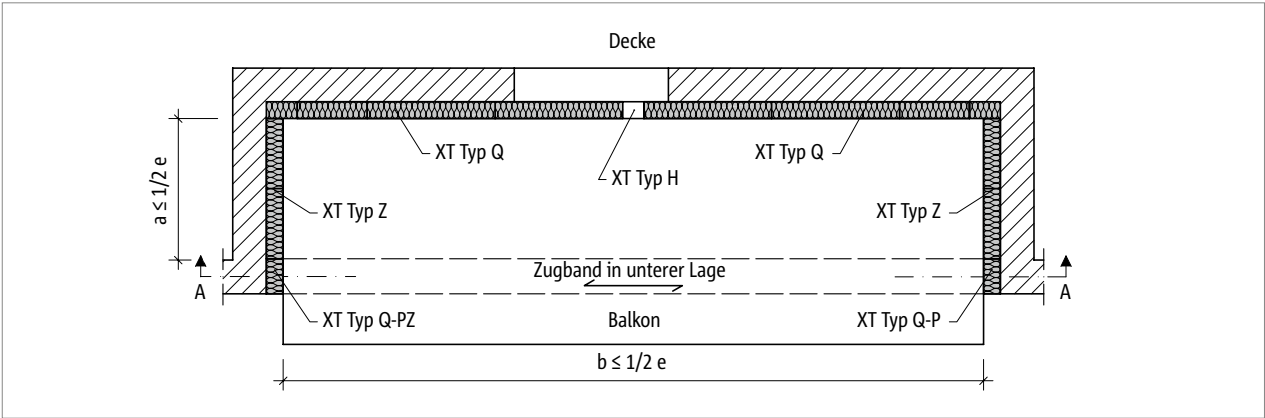
Abb. 208: Schöck Isokorb® T Typ Q-PZ, Q-P: Grundriss Loggia
