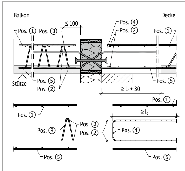
Abb. 198: Schöck Isokorb® XT Typ Q-P-VV5 bis VV16: Bauseitige Bewehrung mit Gitterträger
