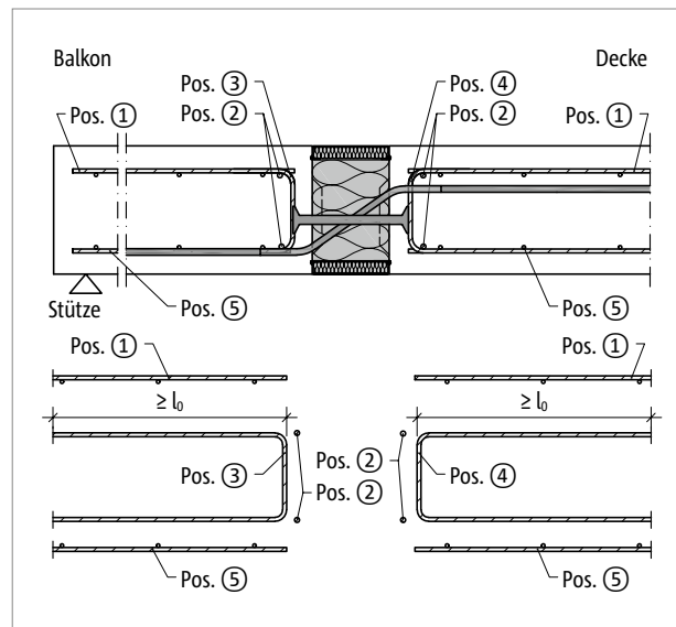
Abb. 201: Schöck Isokorb® XT Typ Q-P-V5 bis V16: Bauseitige Bewehrung
