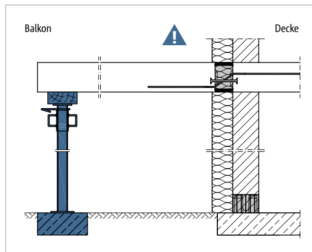
Abb. 217: Schöck Isokorb® XT Typ Q-P: Stützung durchgängig erforderlich
