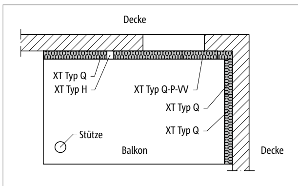
Abb. 177: Schöck Isokorb® XT Typ Q, Q-P-VV: Balkon zweiseitig gelagert mit Stütze und abhebenden Querkraften
