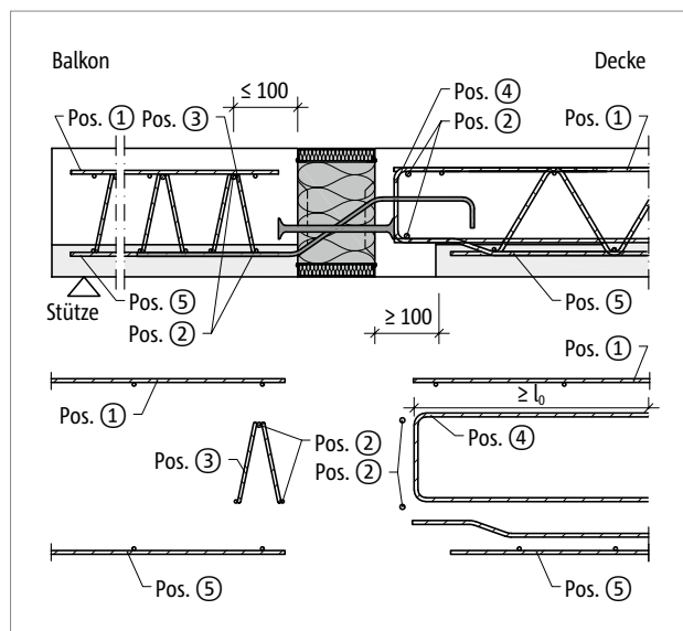
Abb. 202: Schöck Isokorb® XT Typ Q-P-V1 bis V4: Bauseitige Bewehrung mit Gitterträger
