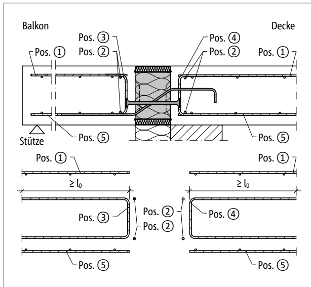
Abb. 194: Schöck Isokorb® XT Typ Q-P-V1 bis V4: Bauseitige Bewehrung
