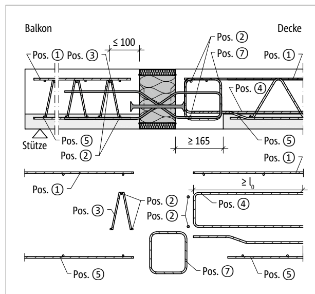
Abb. 203: Schöck Isokorb® XT Typ Q-P-VV1 bis VV4: Bauseitige Bewehrung mit Gitterträger
