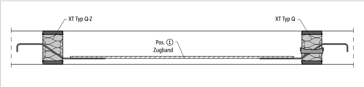
Abb. 168: Schöck Isokorb® XT Typ Q-Z-V1 bis Q-Z-V4, Q-V1 bis Q-V4: Schnitt A-A; einachsig gespannte Stahlbetonplatte
