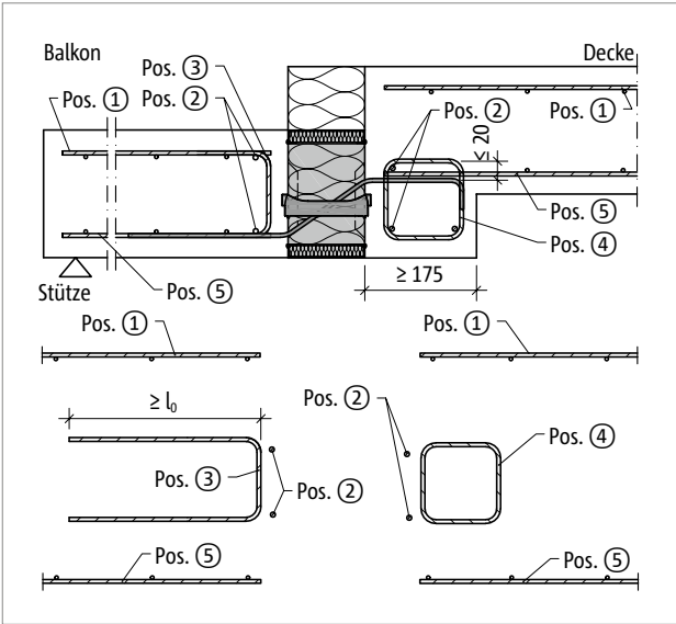
Abb. 165: Schöck Isokorb® XT Typ Q-V1 bis V4: Bauseitige Bewehrung für Balkon mit Höhenversatz nach unten
