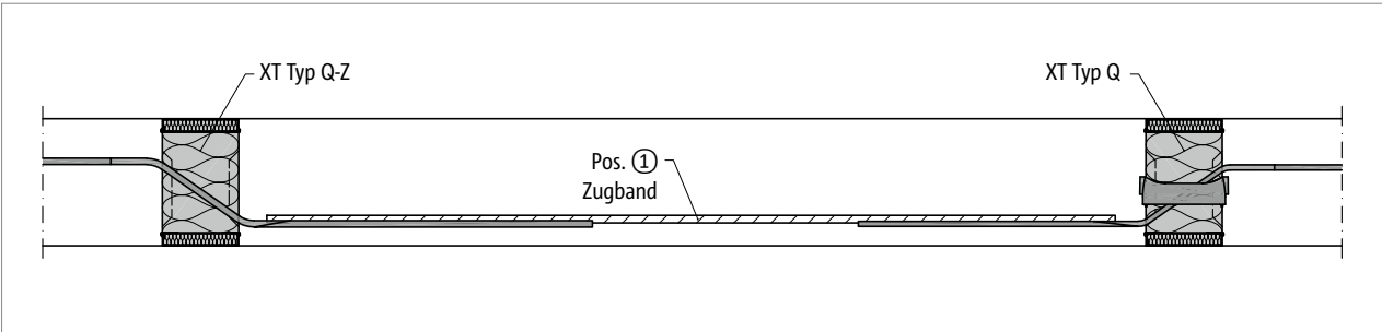
Abb. 169: Schöck Isokorb® XT Typ Q-Z-V5 bis Q-Z-V10, Q-V5 bis Q-V10: Schnitt A-A; einachsig gespannte Stahlbetonplatte
