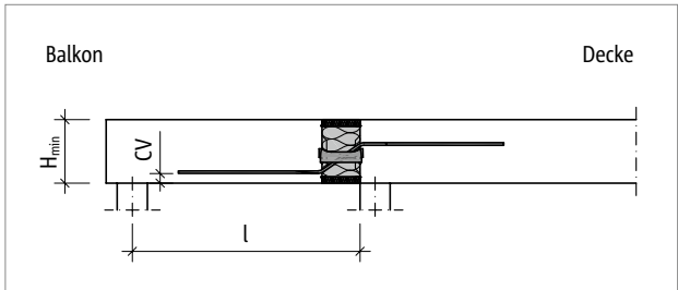
Abb. 143: Schöck Isokorb® XT Typ Q-V5 bis V10: Statisches System
