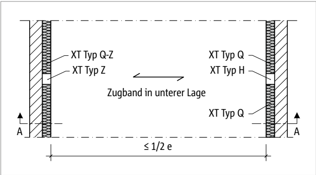
Abb. 167: Schöck Isokorb® XT Typ Q-Z, Q, Z: Einachsig gespannte Stahlbetonplatte
