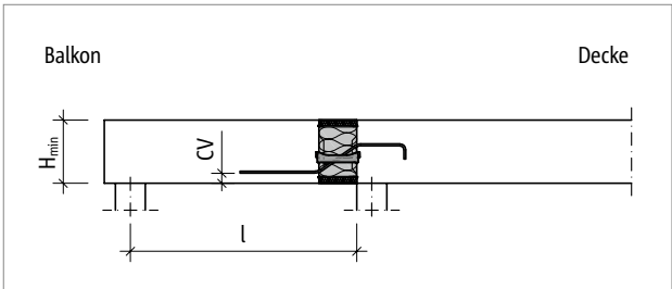
Abb. 142: Schöck Isokorb® XT Typ Q-V1 bis V4: Statisches System
