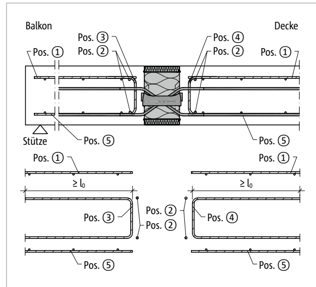
Abb. 158: Schöck Isokorb® XT Typ Q-VV5 bis VV10: Bauseitige Bewehrung
