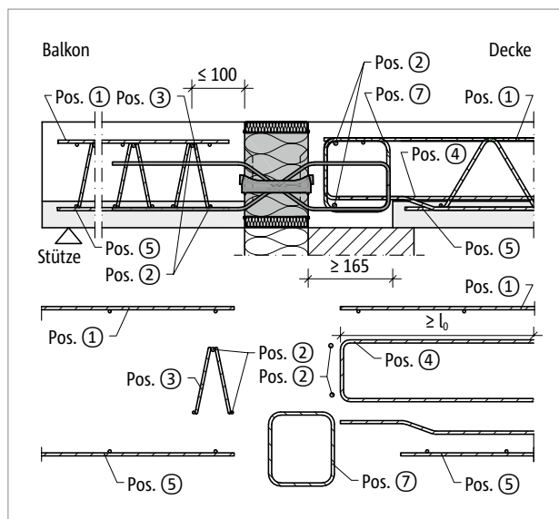
Abb. 154: Schöck Isokorb® XT Typ Q-VV1 bis VV4 Bauseitige Bewehrung mit Gitterträger
