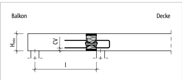
Abb. 145: Schöck Isokorb® XT Typ Q-VV1 bis VV4: Statisches System
