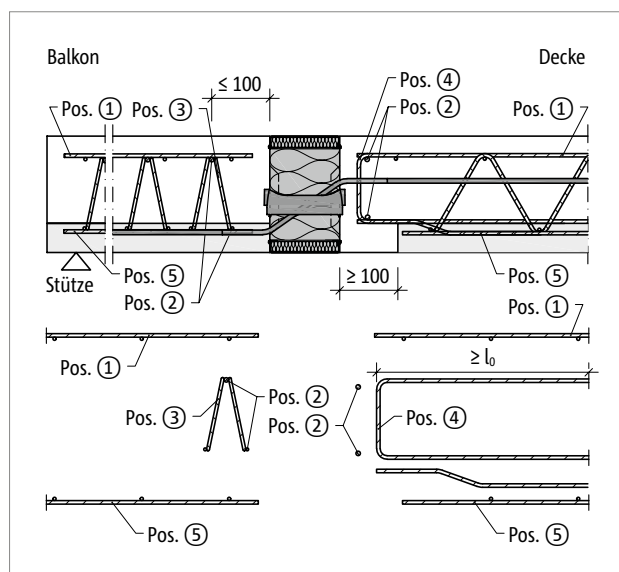
Abb. 163: Schöck Isokorb® XT Typ Q-V5 bis Q-V10: Bauseitige Bewehrung mit Gitterträger
