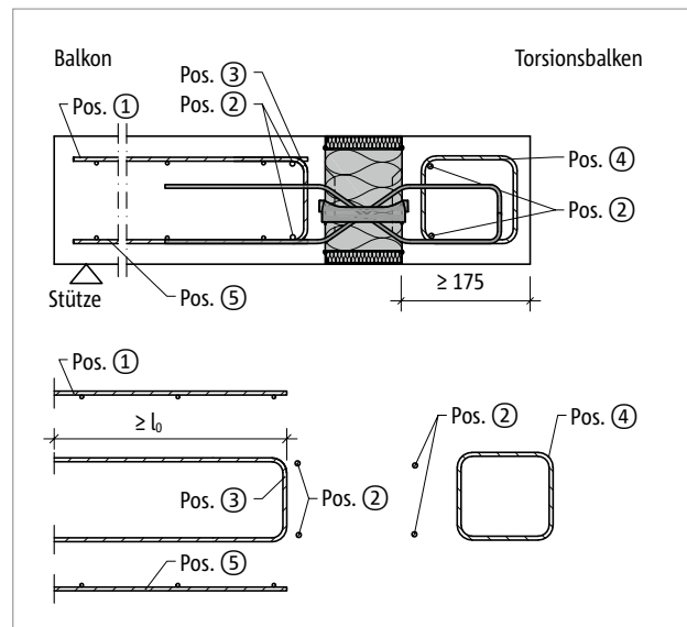
Abb. 160: Schöck Isokorb® XT Typ Q-VV1 bis VV4: Bauseitige Bewehrung in Balken
