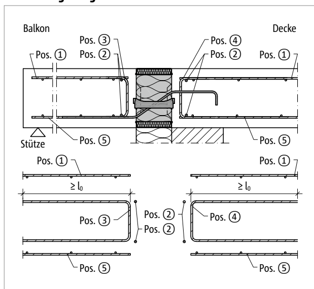
Abb. 151: Schöck Isokorb® XT Typ Q-V1 bis V4 Bauseitige Bewehrung
