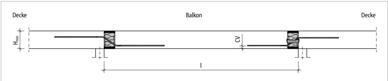
Abb. 144: Schöck Isokorb® XT Typ Q-Z-V5 bis V10, Q-V5 bis V10: Statisches System
