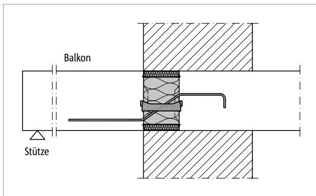
Abb. 137: Schöck Isokorb® XT Typ Q-V1 bis V4: Anschluss bei einschaligem, wärmedämmendem Mauerwerk
