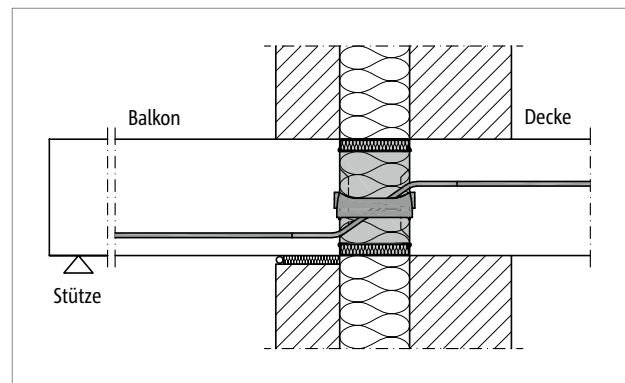
Abb. 138: Schöck Isokorb® XT Typ Q-V5 bis V11: Anschluss bei zweischaligem Mauerwerk mit Kerndämmung
