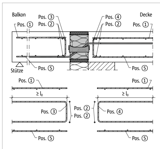
Abb. 152: Schöck Isokorb® XT Typ Q-V5 bis Q-V10: Bauseitige Bewehrung
