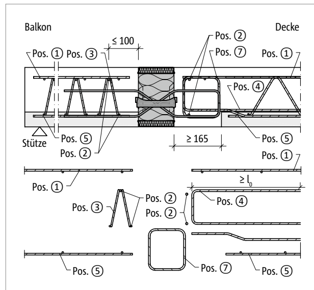
Abb. 162: Schöck Isokorb® XT Typ Q-VV1 bis VV4: Bauseitige Bewehrung mit Gitterträger
