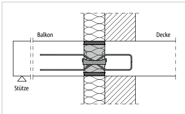
Abb. 139: Schöck Isokorb® XT Typ Q-VV1 bis VV4: Anschluss bei Wärmedämmverbundsystem (WDVS)
