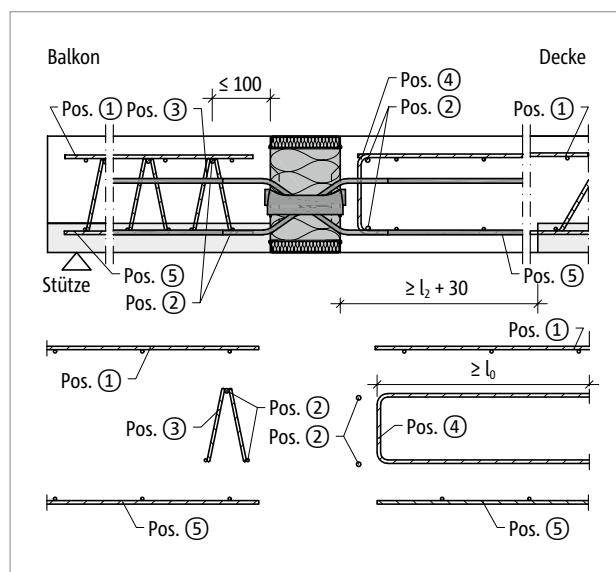
Abb. 164: Schöck Isokorb® XT Typ Q-VV5 bis VV10: Bauseitige Bewehrung mit Gitterträger
