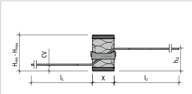
Abb. 150: Schöck Isokorb® XT Typ Q-V5 bis Q-V10: Produktschnitt
