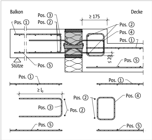
Abb. 166: Schöck Isokorb® XT Typ Q-VV1 bis VV4: Bauseitige Bewehrung für Balkon mit Höhenversatz nach oben
