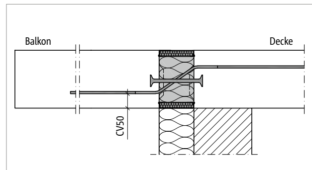
Abb. 173: Schöck Isokorb® XT Typ Q-P-CV50: Schnitt
