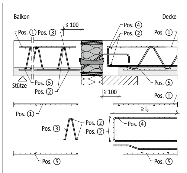
Abb. 153: Schöck Isokorb® XT Typ Q-V1 bis V4 Bauseitige Bewehrung mit Gitterträger
