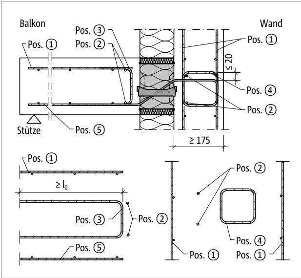
Abb. 156: Schöck Isokorb® XT Typ Q-V1 bis V4: Bauseitige Bewehrung in Wand
