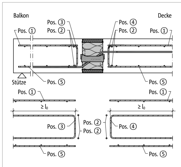
Abb. 159: Schöck Isokorb® XT Typ Q-V5 bis Q-V10: Bauseitige Bewehrung
