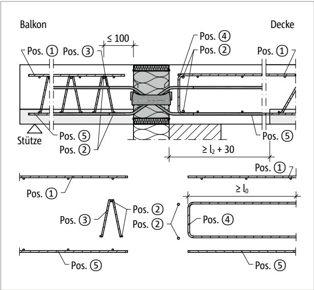
Abb. 155: Schöck Isokorb® XT Typ Q-VV5 bis VV10 Bauseitige Bewehrung mit Gitterträger
