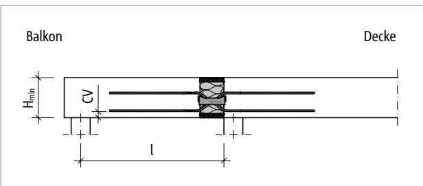
Abb. 146: Schöck Isokorb® XT Typ Q-VV5 bis VV10: Statisches System
