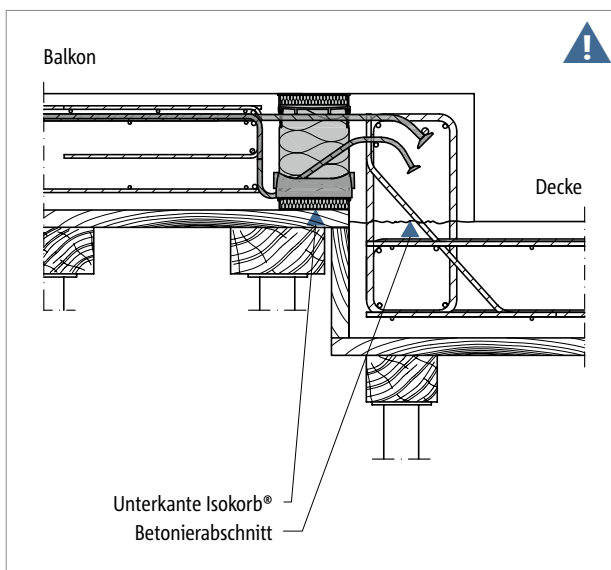
Abb. 121: Schöck Isokorb® XT Typ K-O: Ortbetonbalkon mit Höhenversatz nach oben
