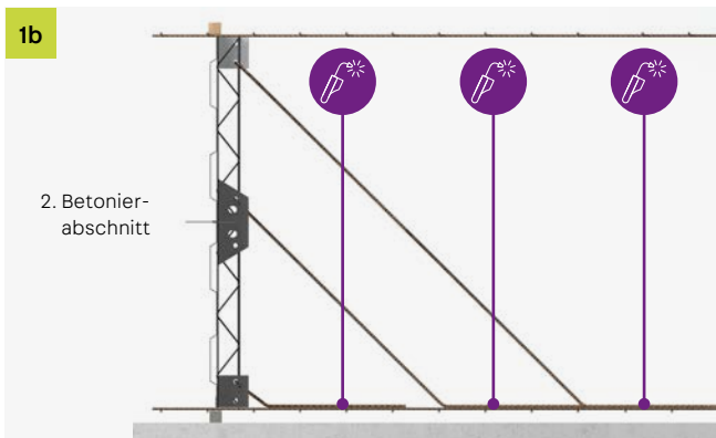
Schematischer Querschnitt der Einbausituation
