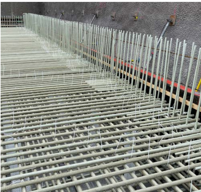
Bewehrung der Bodenplatte, Wände und Decke des Kryostaten- raums, Paul Scherrer Institut (PSI), Villigen, Schweiz
