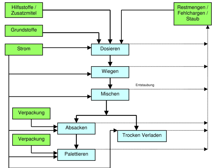
Graphik 1: Herstellungsprozess (grün: Input; blau: Einheitsprozess)
