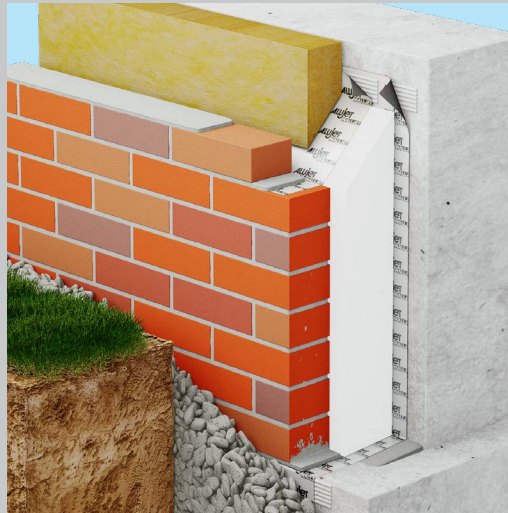
Im zweischaligen Mauerwerk auf Beton
