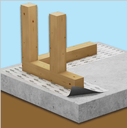
Als Abdichtungsbahn im Holzrahmenbau
