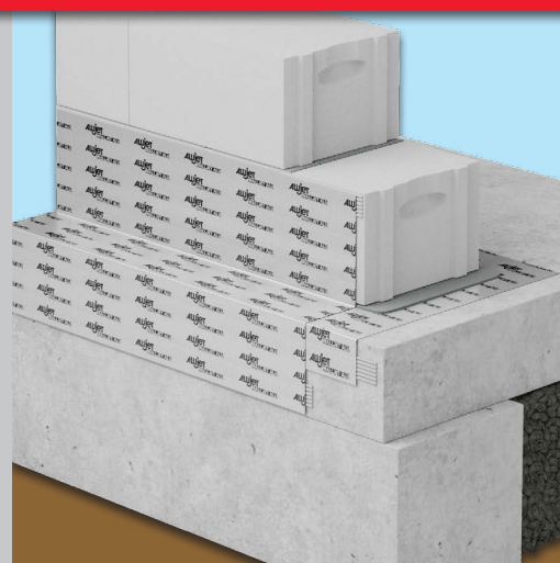
Im einschaligen Mauerwerk als Sockelabdichtung
