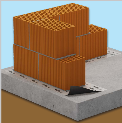
Im einschaligen Mauerwerk auf der Bodenplatte
