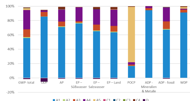
Abbildung: Einfluss der Lebenswegphasen auf die Umweltwirkungen für Haftvermittler auf Dispersionsbasis
