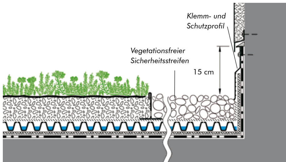
Bei begrünten Dächern sind die Anschlußbereiche vegetationsfrei zu halten und die Abdichtung ist am Wandanschluß zu schützen.
