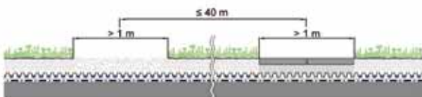
Mindestens alle 40 m ein Streifen aus Kies, Zincolit® oder Betonplatten
