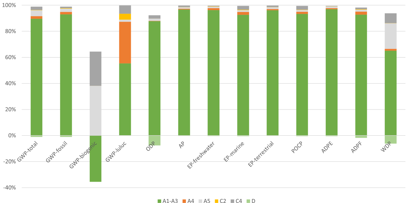
Relative Beiträge der verschiedenen Lebenszyklusphasen von Steinwolle mit mittlerer Rohdichte
