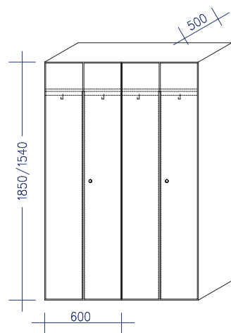
Schwarz-Weiß-Schrank zur Trennung von Arbeits- und Straßenkleidung 2-türig, SWM2
