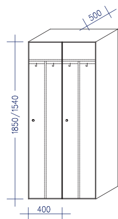
Schwarz-Weiß-Schrank zur Trennung von Arbeits- und Straßenkleidung 1-türig, SWM1
