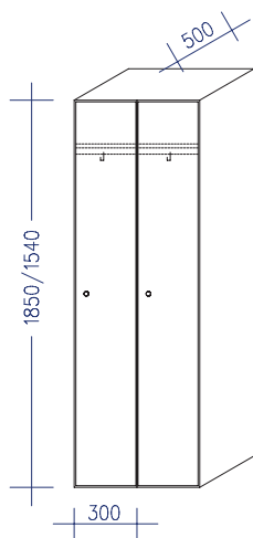
Garderobenschrank 1-türig, GM1
