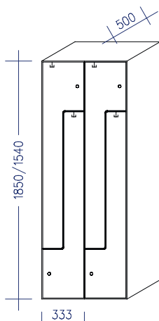
Z-Garderobenschränk GHZ
