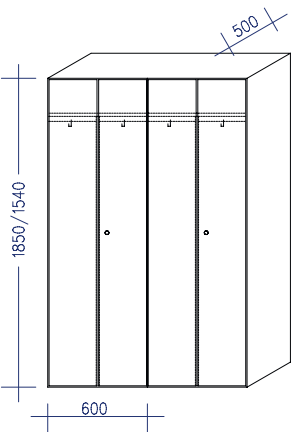
Schwarz-Weiß-Schrank zur Trennung von Arbeits- und Straßenkleidung 2-türig, SWH2
