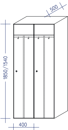
Schwarz-Weiß-Schrank zur Trennung von Arbeits- und Straßenkleidung 1-türig, SWH1
