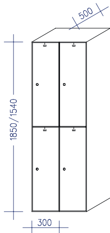
Garderobenschränk 1/2-türig, GH2
