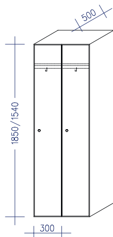
Garderobenschrank 1-türig, GH1
