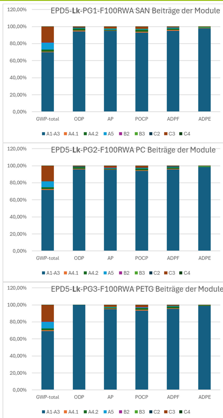
Abbildung 2: Prozentuale Anteile der Module an ausgewählten Umweltwirkungsindikatoren
