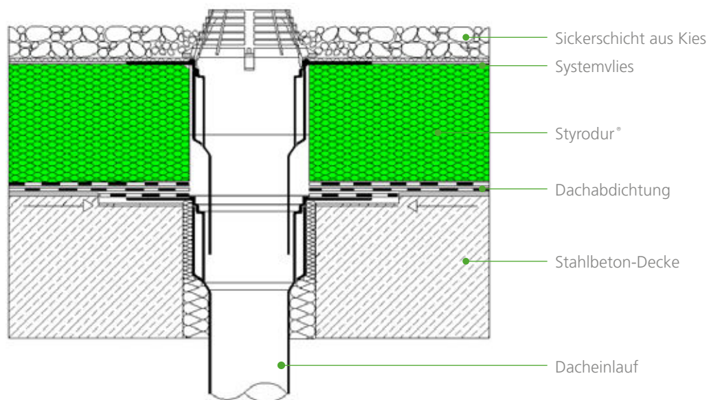
Abb. 6: Dacheinlauf mit zwei Entwässerungsebenen für die Entwässerung der Dachfläche auf und unter der Dämmschicht.
