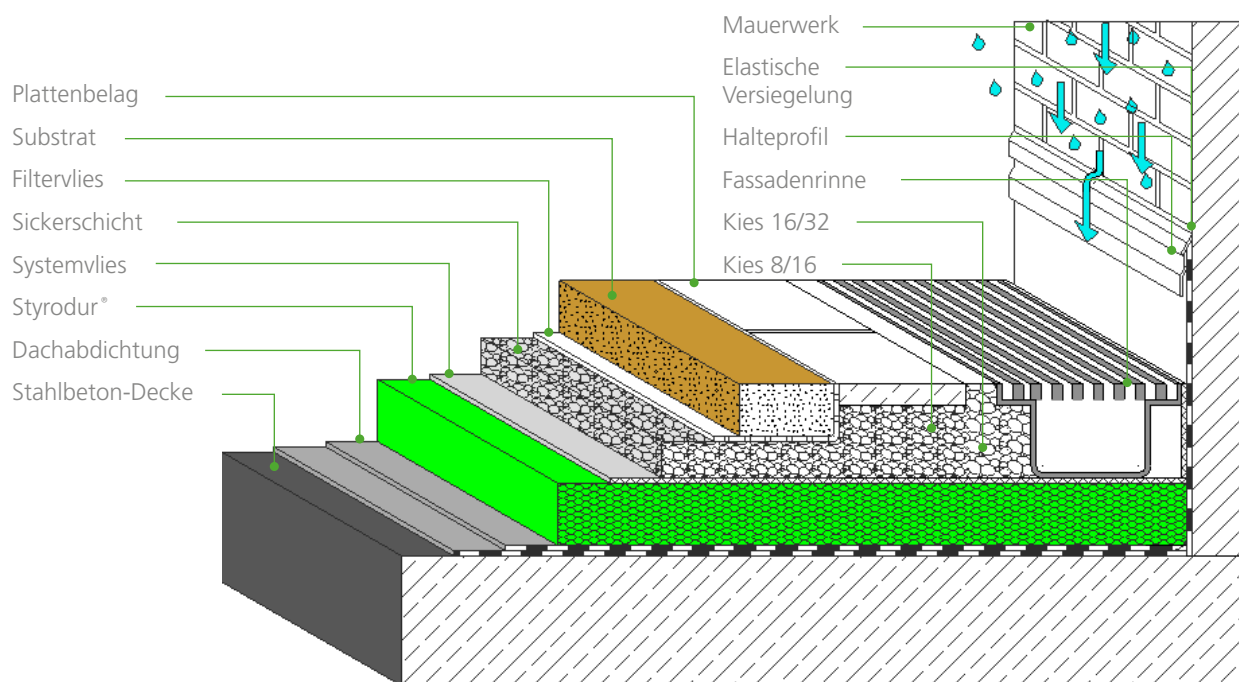
Abb. 31: Anschluss UK-Gründach an eine aufgehende Wand mit Fassadenrinne.
