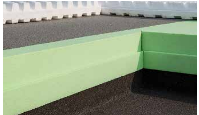
Abb. 20: Styropor-Formteilplatten zur Wasserrückhaltung und Drainage eines begrünten Umkehrdaches mit Styrodur®.
