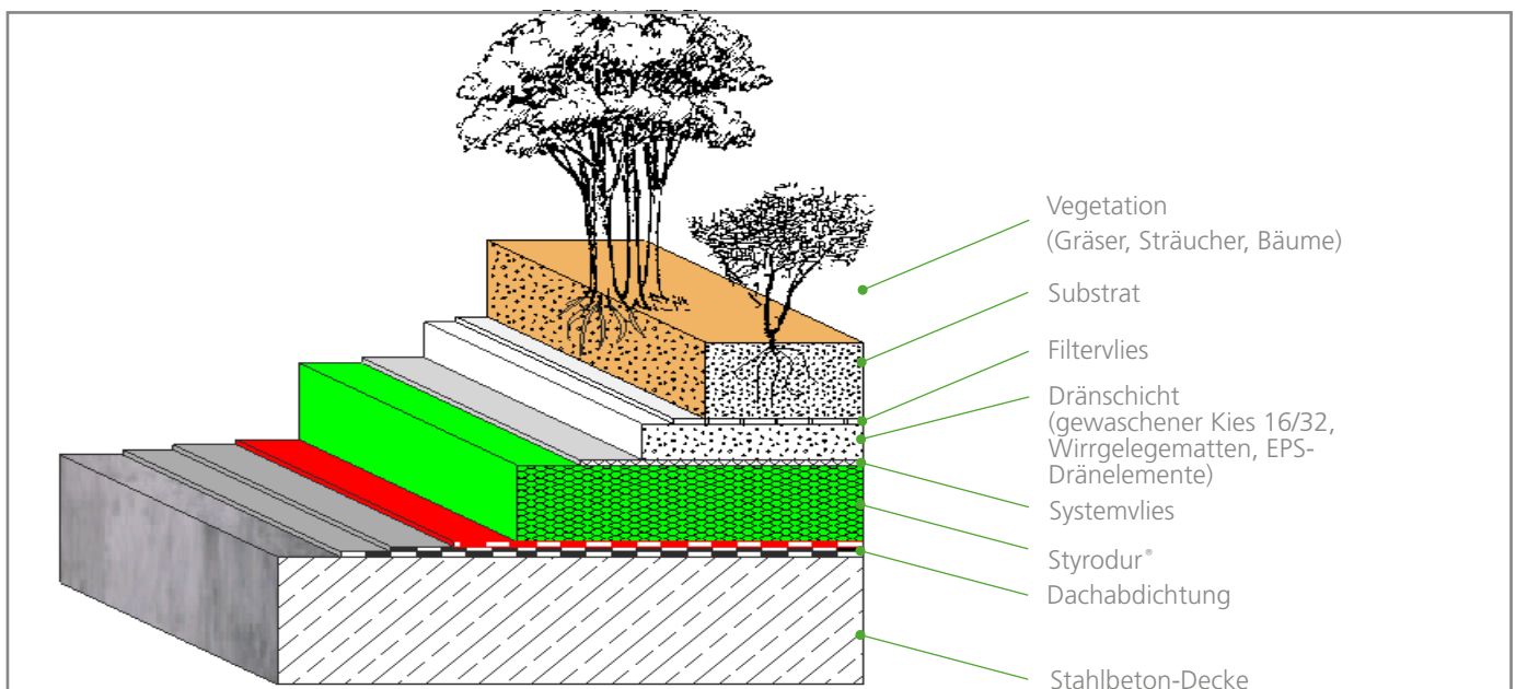
Abb. 26: Schnitt durch ein intensiv begrüntes Umkehrdach.
