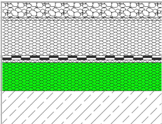
Abb. 12: Ausführung des Duodachs mit Kiesschüttung.
