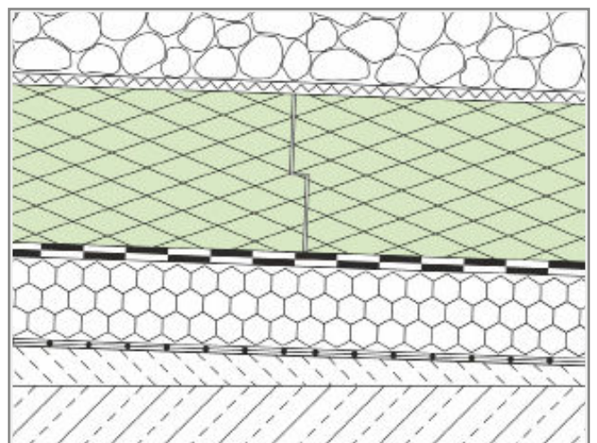
Abb. 16: Saniertes Plusdach mit Gefälledämmung im Altbestand.
