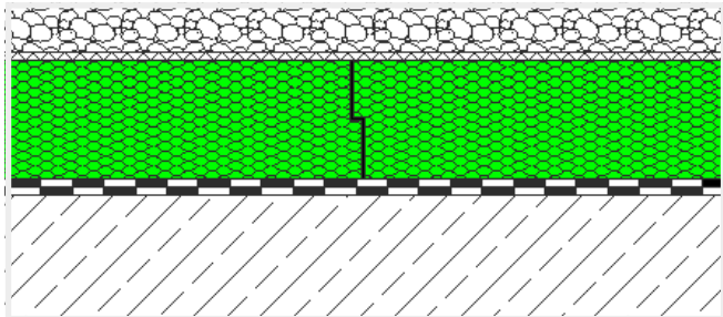
Abb. 9: Ausführung einlagig bekiestes Umkehrdach.
