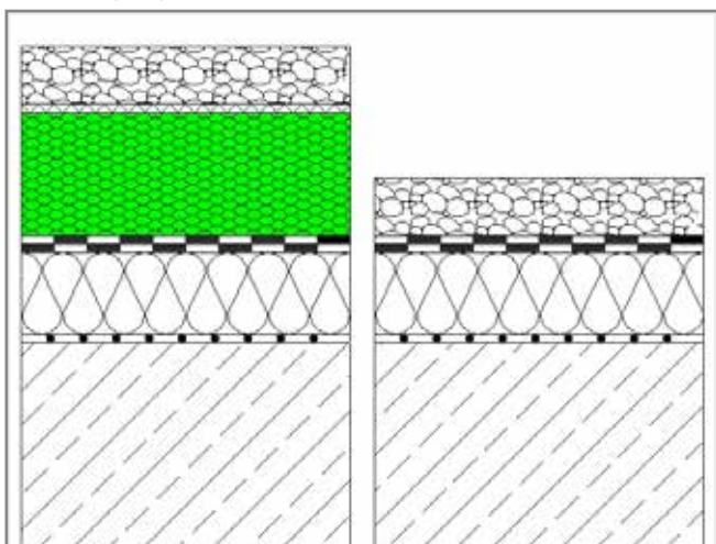
Abb. 15: Links neuer Zustand eines Plusdaches, rechts alter Zustand des Warmdaches.
