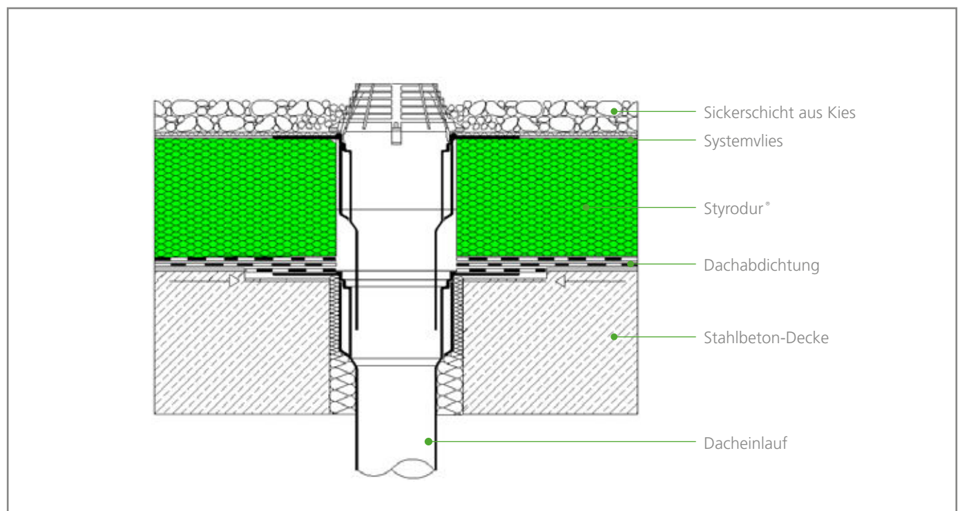
Abb. 6: Dacheinlauf mit zwei Entwässerungsebenen für die Entwässerung der Dachfläche auf und unter der Dämmschicht.
