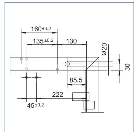
Anschlagmaße Linkstür
