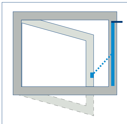
Drehflügel DIN R AUSWÄRTS (Antrieb nicht schwenkbar) Kabelaustritt immer nach oben!
