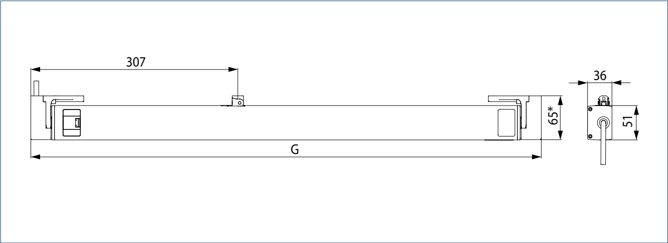
G = Länge | * = Konsolensatz A
