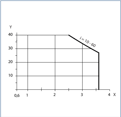
X = Gesamtflügelbreite (Summe aller Flügelbreiten) [m] | Y = Füllgewicht [kg/m²]
