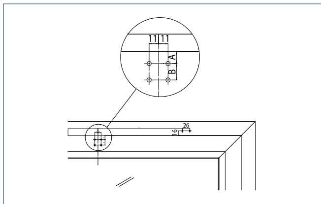
Rahmenmontage EINWÄRTS
