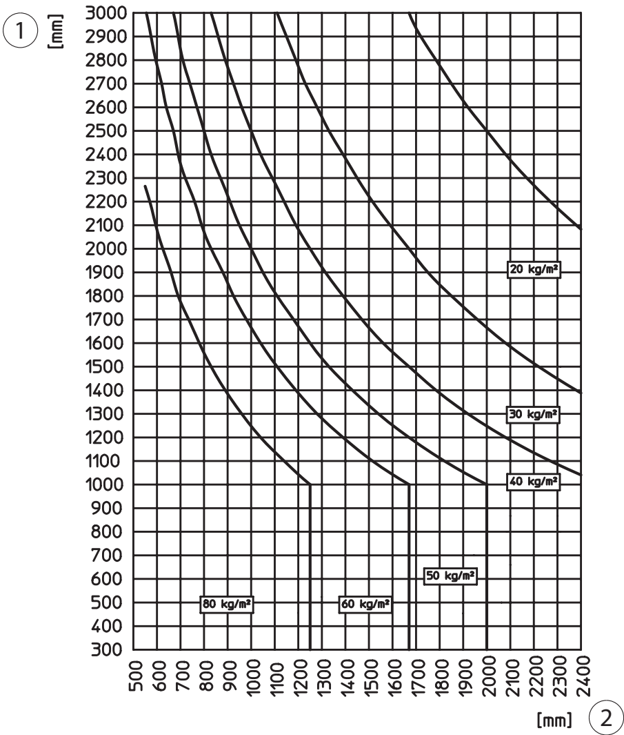
1 = Flügelhöhe | 2 = Flügelbreite
