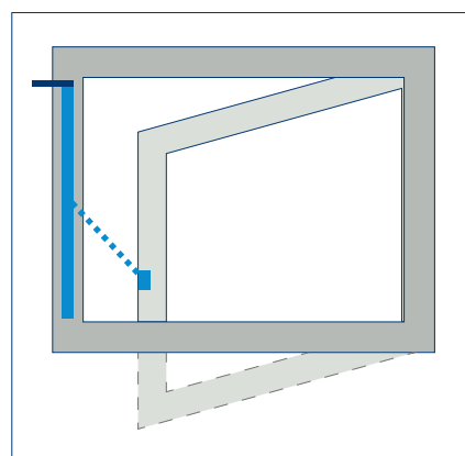
Drehflügel DIN L AUSWÄRTS (Antrieb nicht schwenkbar)
