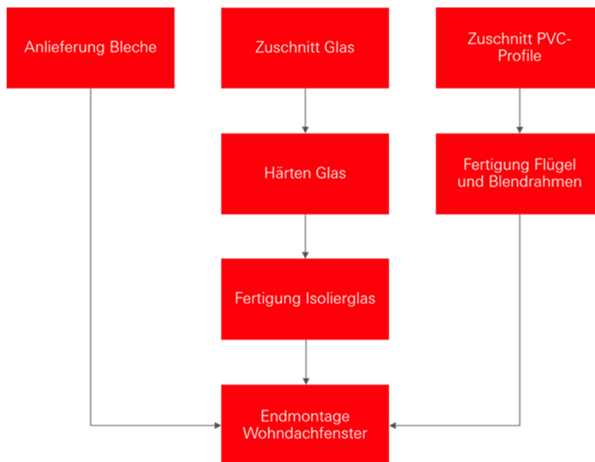
Abbildung 1 Produktherstellung Kunststofffenster
