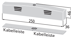
Standard-Abdeckung RZO 02 für Rauchschalzentrale RSZ 142
