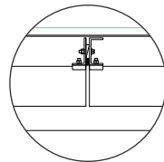
Verdeckter Pfosten an einer Verbindungsstelle zwischen zwei Lamellen
