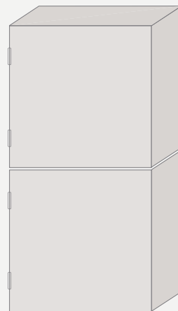
Korpus (BxHxT) 1 1060 x 2080 x 1060 mm 2 3180 x 2080 x 1060 mm
