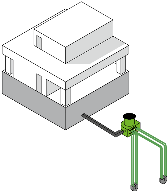
Abb. 03-1 Erdwärmesonde
