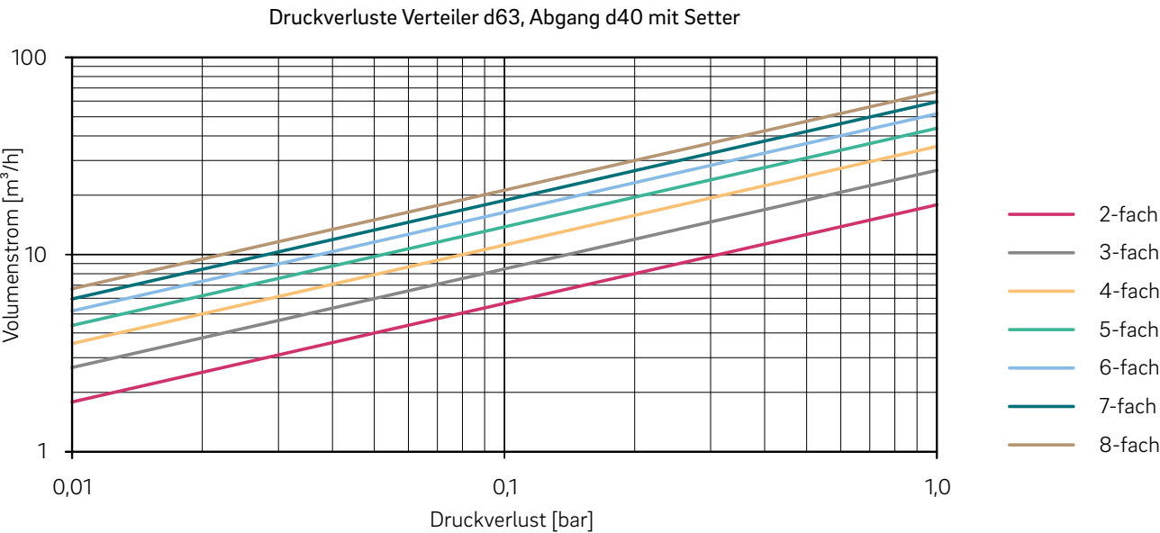
Abb. 07-4 Diagramm Druckverlust Verteiler d63, Abgang d40 mit Setter
