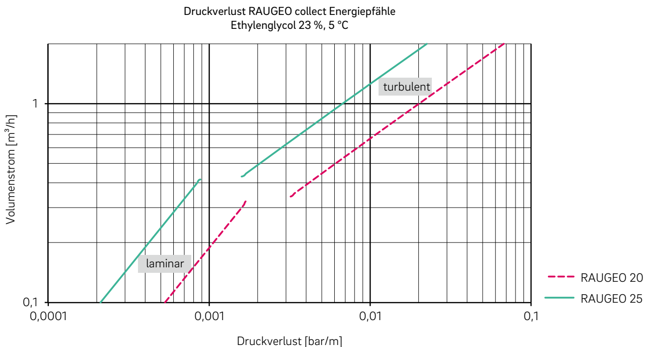
Abb. 06-1 Diagramm Druckverlust RAUGEO collect Energiepfähle
