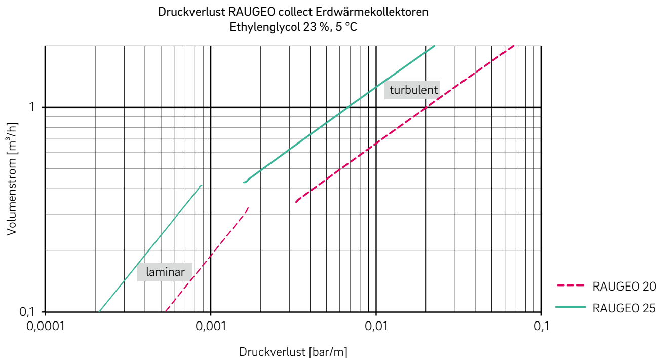
Abb. 05-1 Diagramm Druckverlust RAUGEO collect Erdwärmekollektoren
