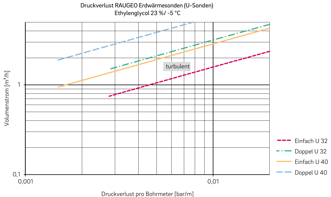
Abb. 04-1 Diagramm Druckverlust U-Sonden
