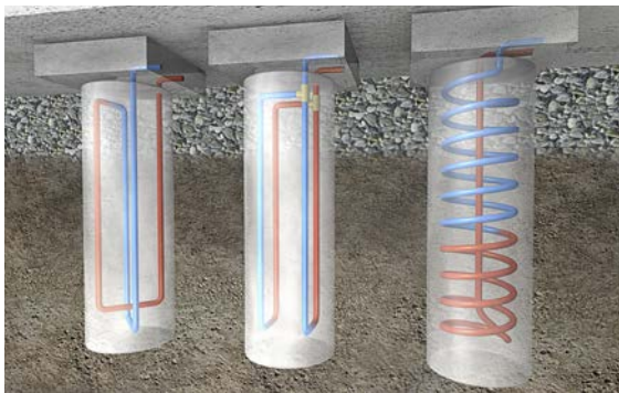
Abb. 06-2 Kollektorröhre im Bewehrungskorb
