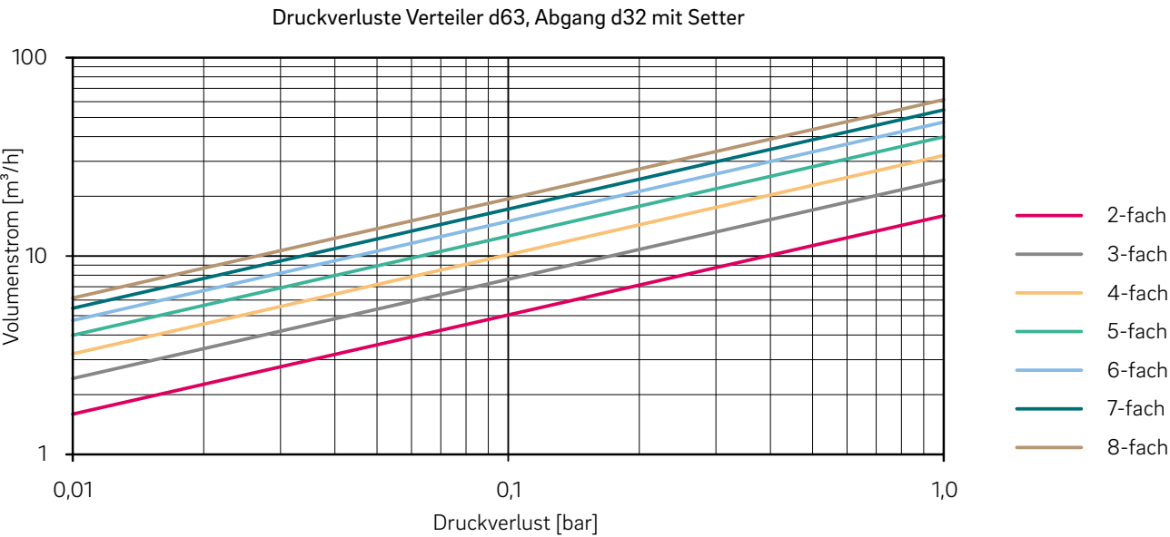
Abb. 07-3 Diagramm Druckverlust Verteiler d63, Abgang d32 mit Setter
