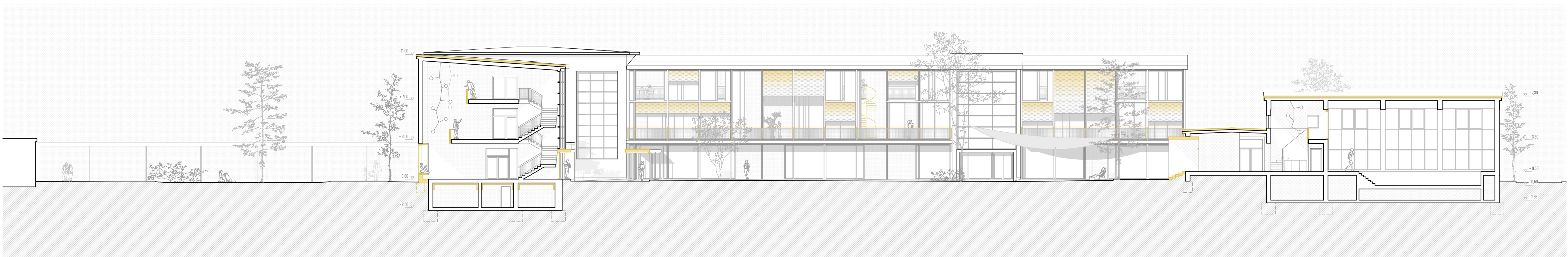
Ansicht Ost
