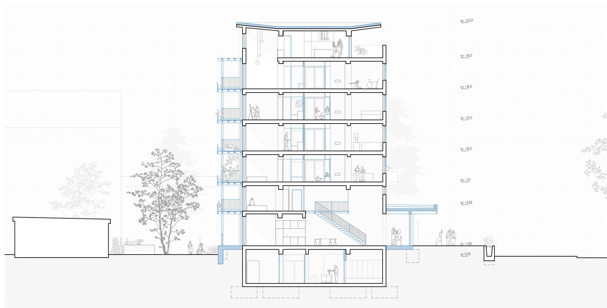
Schnitt A-A
