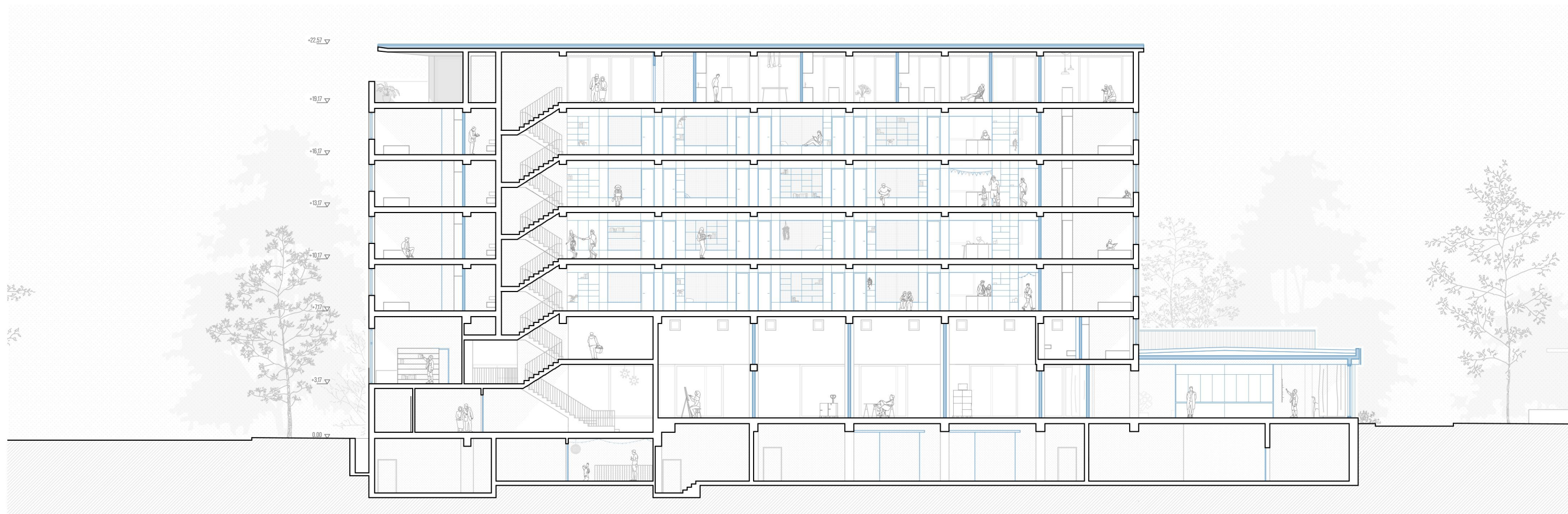
Schnitt B-B
