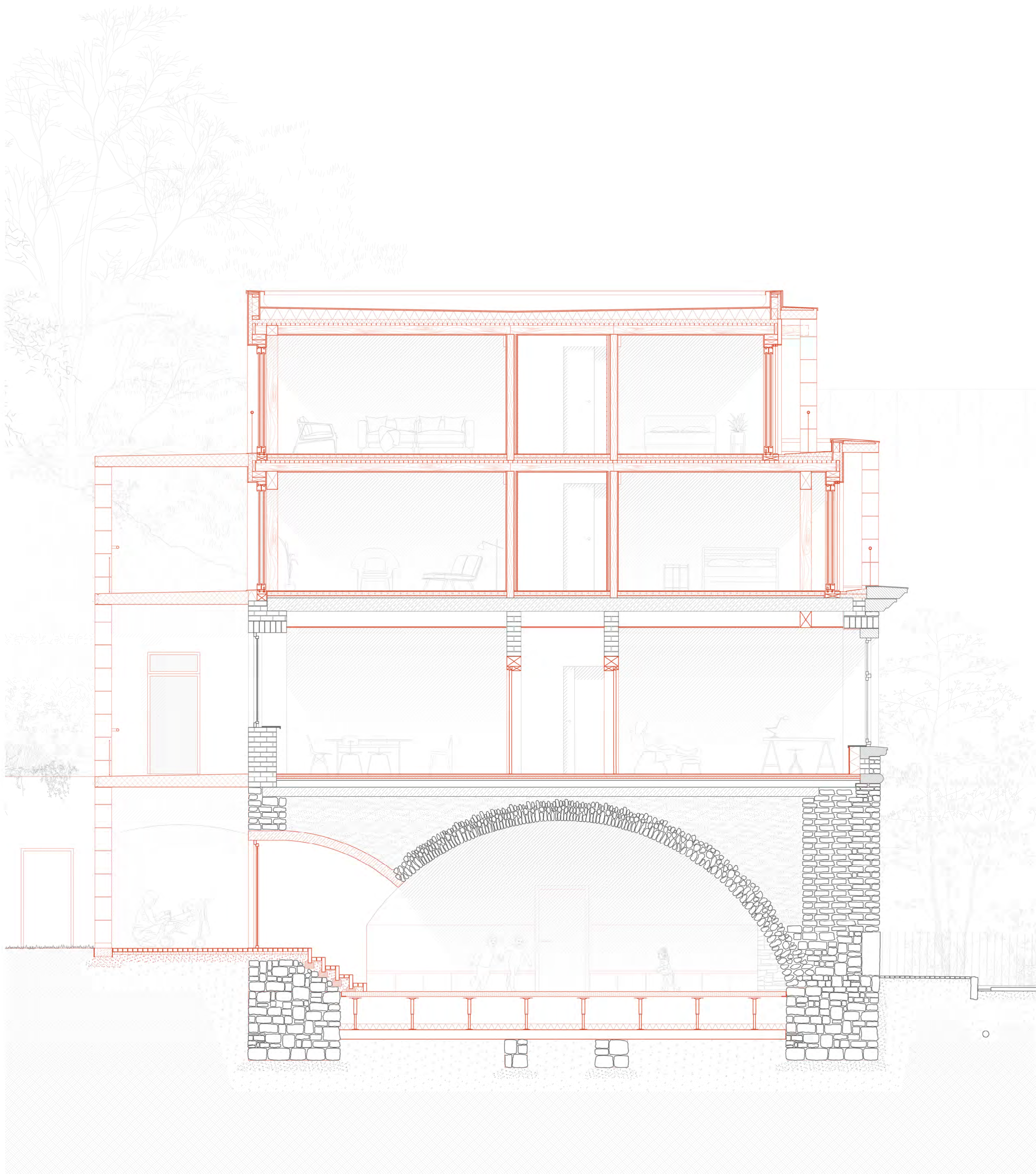
Konstruktionsschnitt M 1 : 50
