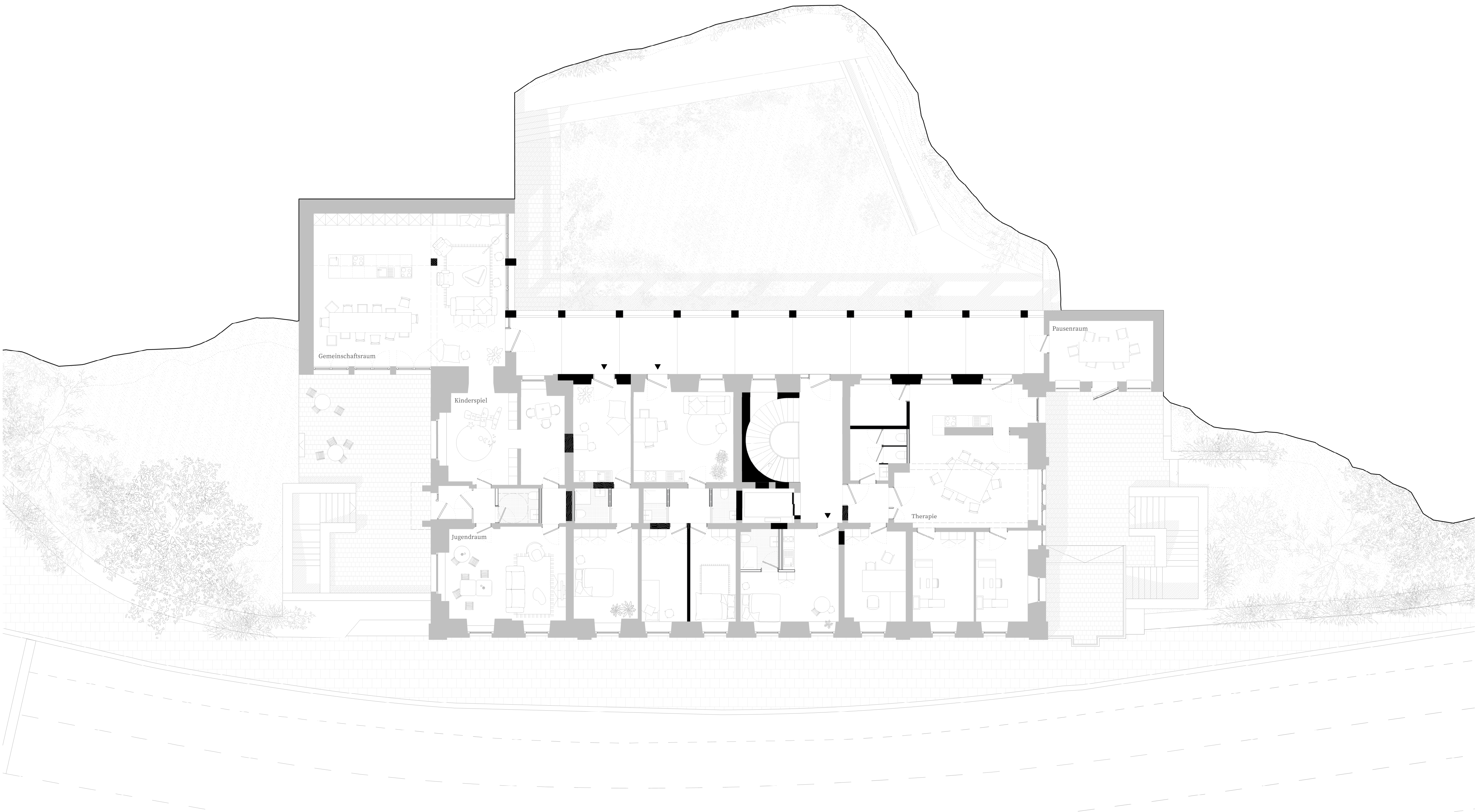
Grundriss 1. Obergeschoss M 1 : 100
