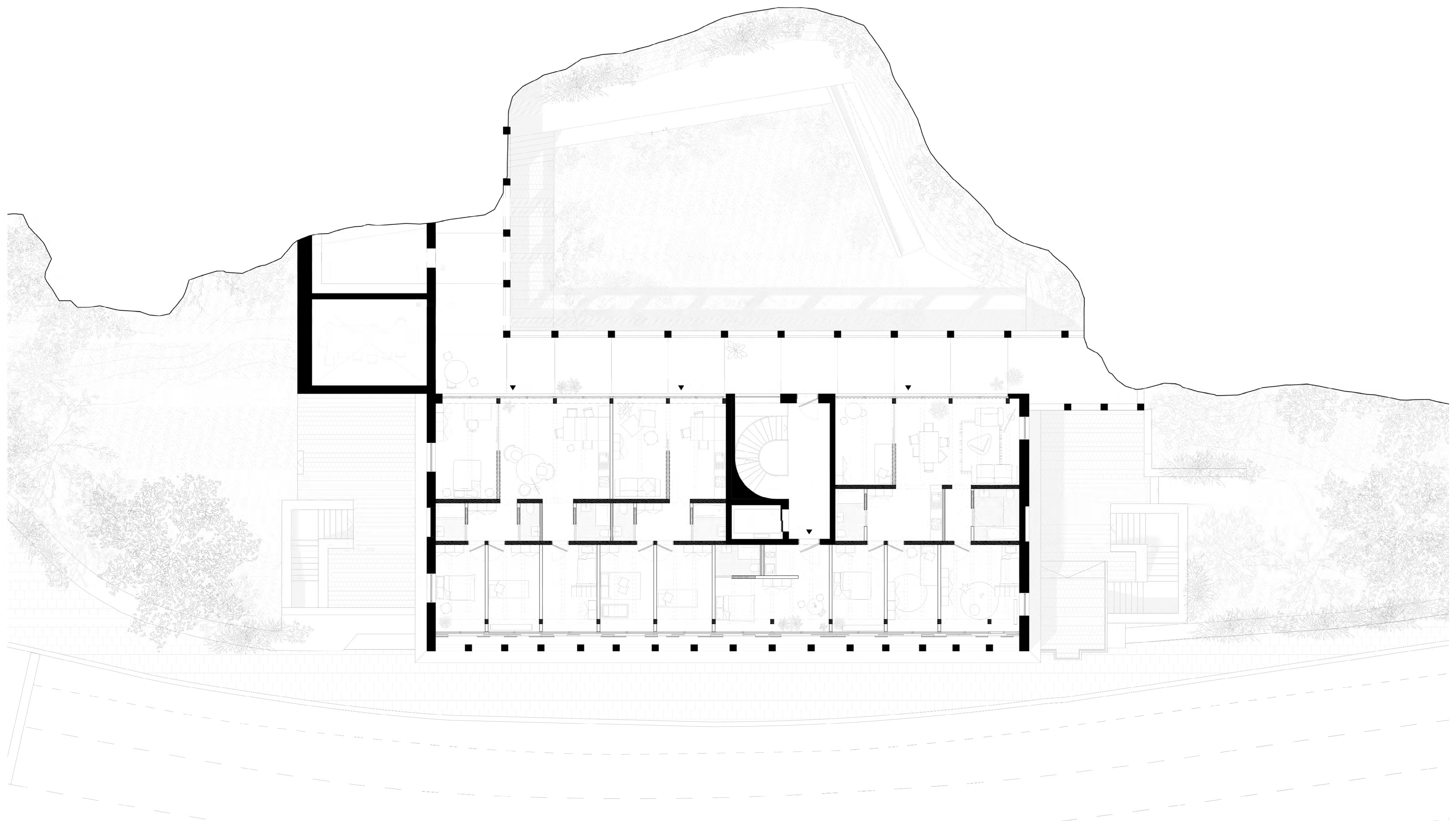
Grundriss 2. Obergeschoss M 1 : 100
