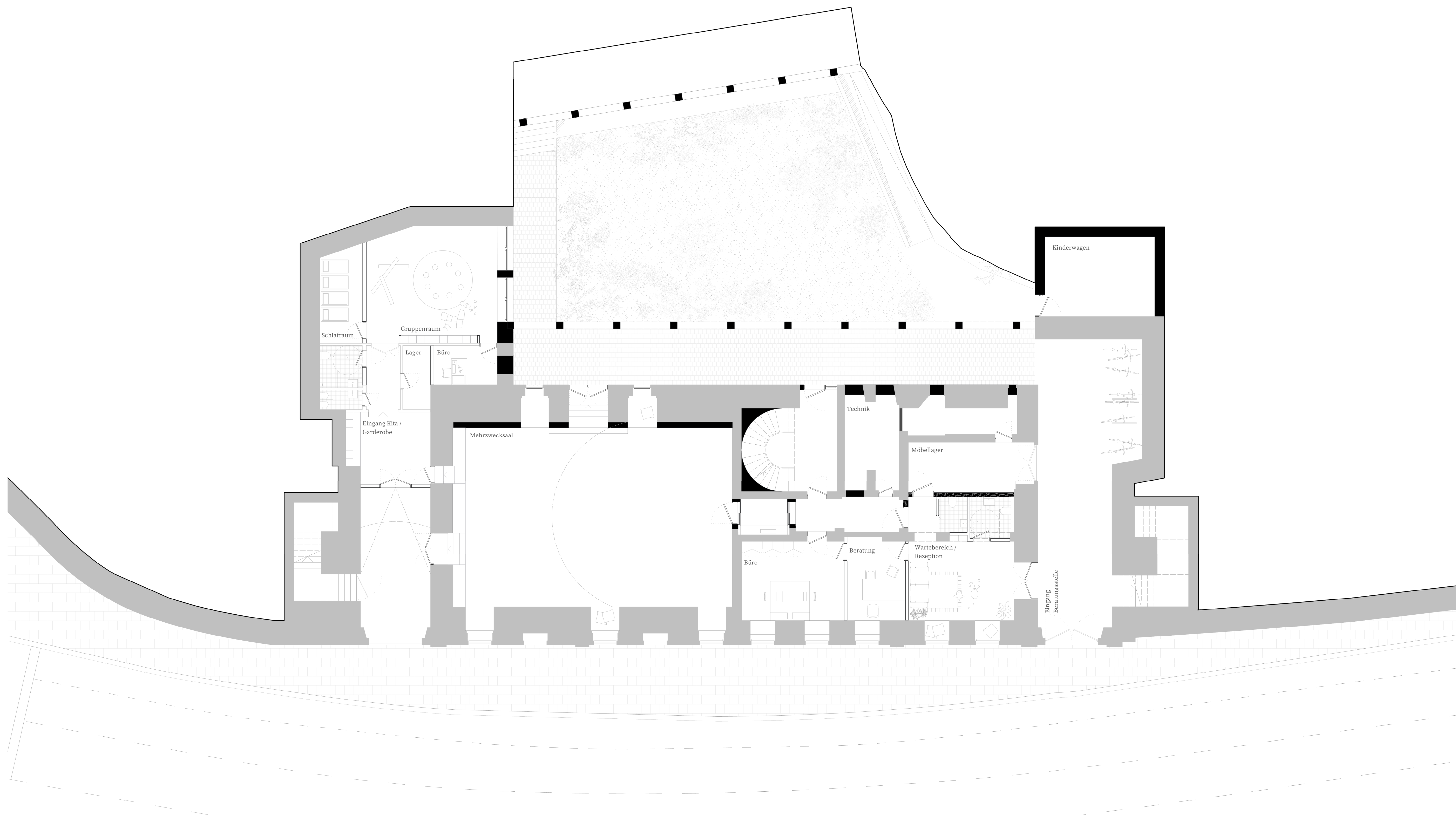
Grundriss Erdgeschoss M 1 : 100
