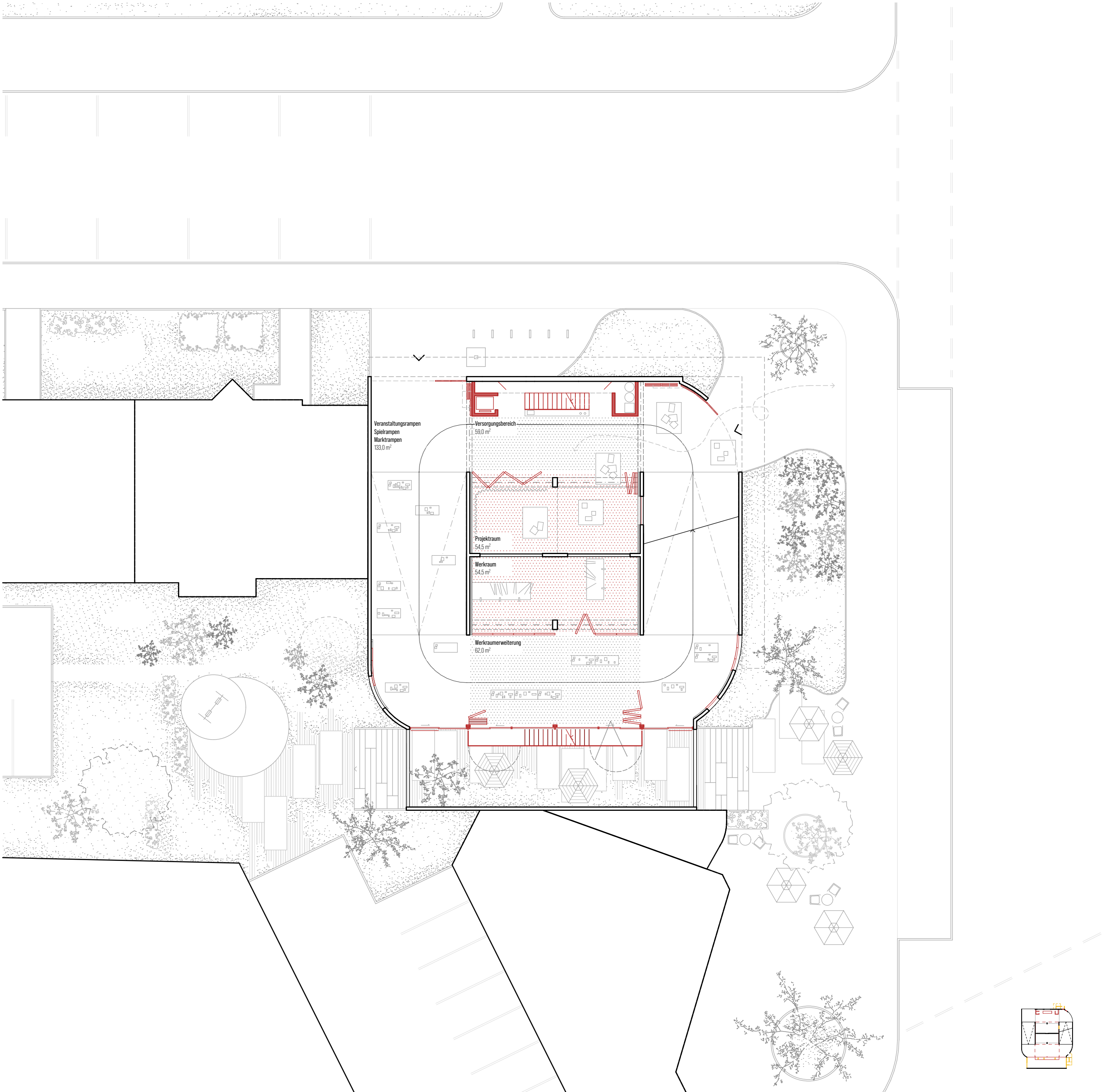
Grundriss Erdgeschoss 1:200
