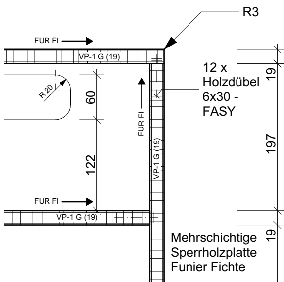
DETAILSCHNITT 1:5
