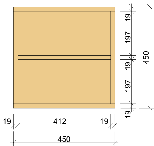
VORDERANSICHT 1:10
