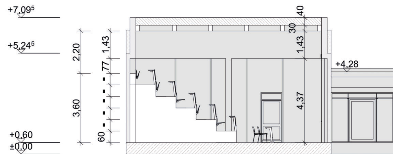
Schnitt E-E
