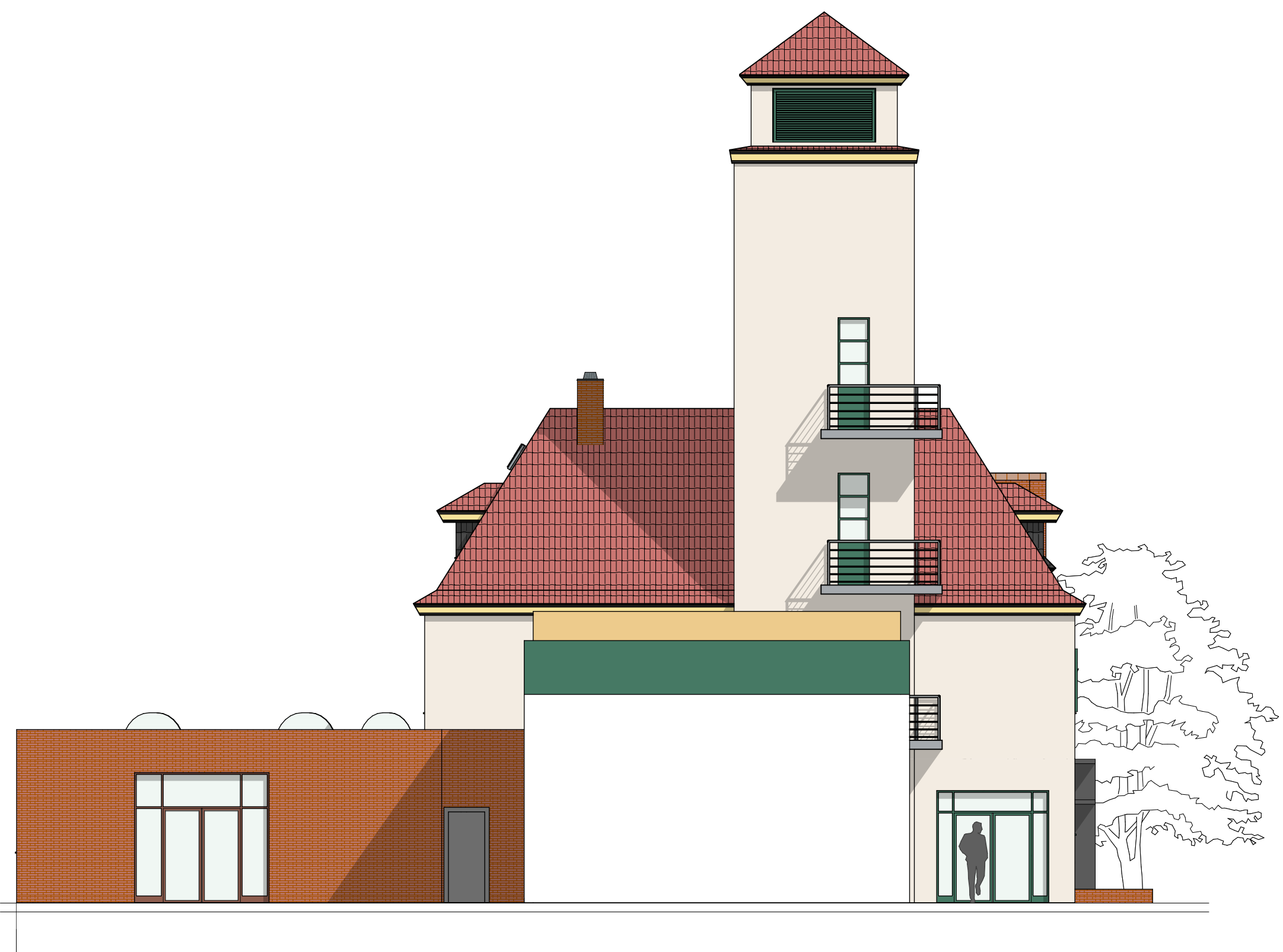
Ansicht Nord
