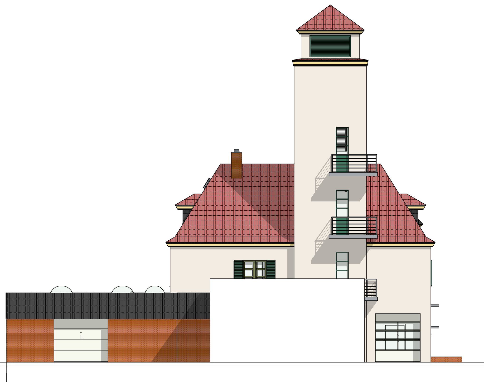
Ansicht Nord
