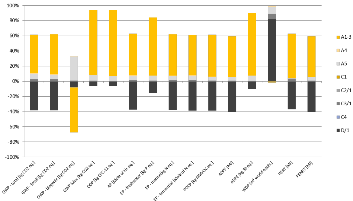
Relative Beiträge der Module zu Umweltwirkungen und Primärenergieeinsatz von 1 m 2 Sikaplan® G-15 (100 % stoffliches Recycling)
