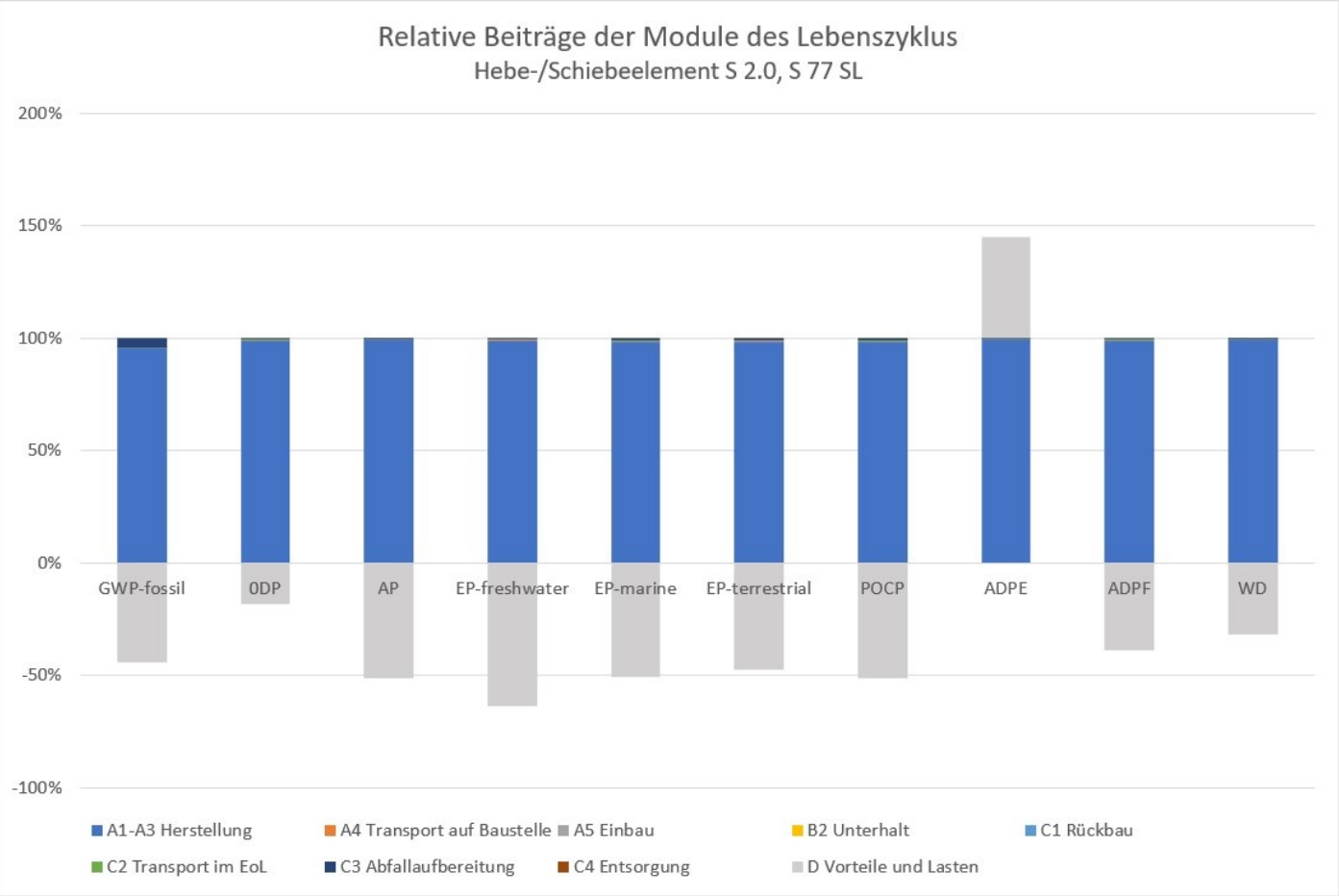
Abbildung 1: Umweltauswirkungen des heroal Hebe-/Schiebeelement S 77 SL über seinen gesamten Lebenszyklus (normiert an den Auswirkungen des Produktlebenszyklus A1-C4 = 100 %) Die Ökobilanz für das heroal Hebe-/Schiebeelement S 77 SL wird von der Herstellung (Module A1-A3) sowie von den Belastungen und Vorteilen außerhalb des Produktsystems (Modul D) dominiert, die sich aus dem Recycling oder der energetischen Verwertung am Ende der Lebensdauer ergeben. Alle anderen Module sind von untergeordneter Bedeutung. Dies liegt daran, dass die Module A1-A3 sowohl die Auswirkungen bei heroal hinsichtlich der Materialzusammensetzung als auch der Transport des vorkonfektionierten Produkts um Metallbauer sowie die Umweltwirkungen beim Metallbauer umfassen. Die Auswirkungen 'ab Werkstor' – also der verbleibende Transport zur Baustelle sowie die manuelle Montage, die jährliche Reinigung und das Ende der Lebensdauer – sind hingegen
